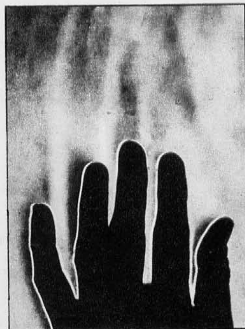
ШЛИРЕН-МЕТОД ВЫЯВЛЯЕТ ТЕПЛОВЫЕ ПОТОКИ ВОЗДУХА, ИДУЩИЕ ВВЕРХ ОТ ПАЛЬЦЕВ. ЭТОТ МЕТОД ШИРОКО ИСПОЛЬЗУЕТСЯ ДЛЯ ИССЛЕДОВАНИЯ САМЫХ РАЗЛИЧНЫХ ПОТОКОВ, НАПРИМЕР В АЭРОДИНАМИЧЕСКИХ ТРУБАХ ПРИ ИСПЫТАНИЯХ МАКЕТОВ САМОЛЕТОВ. УИЛЬЯМ РЕЙД , 1950
